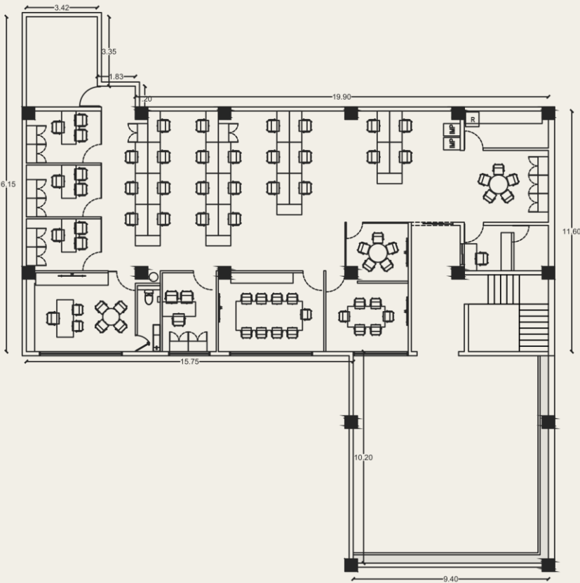
Plantas arquitectónicas originales sin fondo
