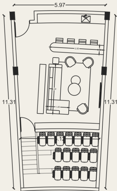
PLANTA ARQUITECTÓNICA
